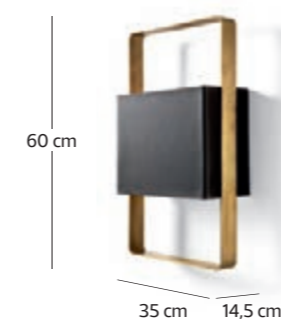
art. Contessa A35 2 x max 53 W E27
