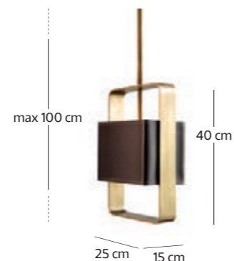
art. Contessa S30 1 x max 53 W E27
