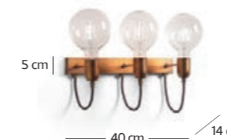
art. Bolle BLL/A3 3 x max 42 W E27
