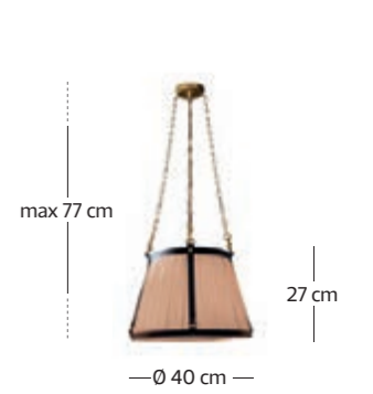
art. Selleria S 40 IN 1 x max 42 W E27
