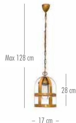
Titty Out S 17 1 x E 27 Max 42W IP 43 ⚡ CE F
